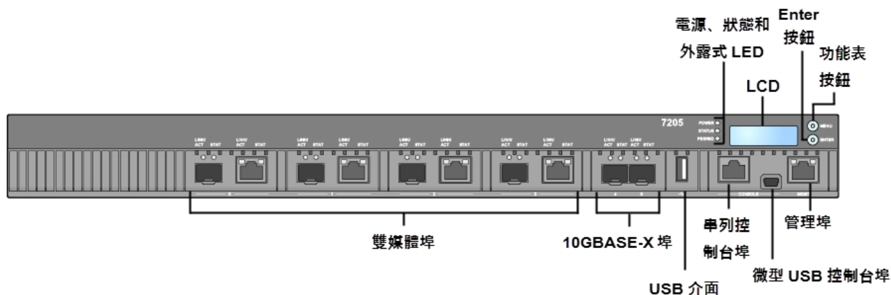
圖 2: W-7205 控制器的後置面板
