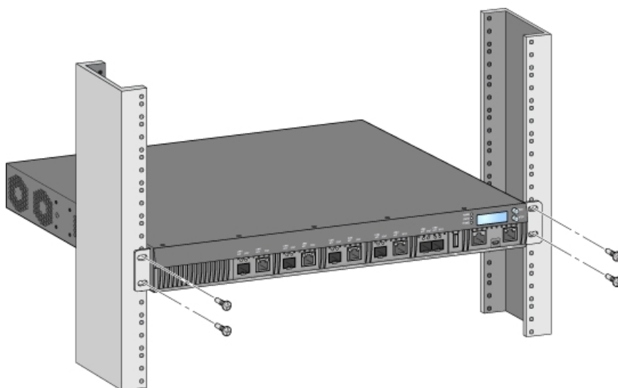
圖 8: 前機架安裝
