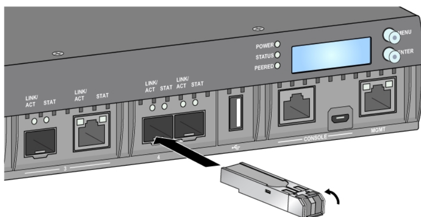
圖 14: 安裝 SFP 模組
