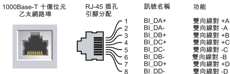
圖 3: 10/100/1000BASE-T 埠引出線
