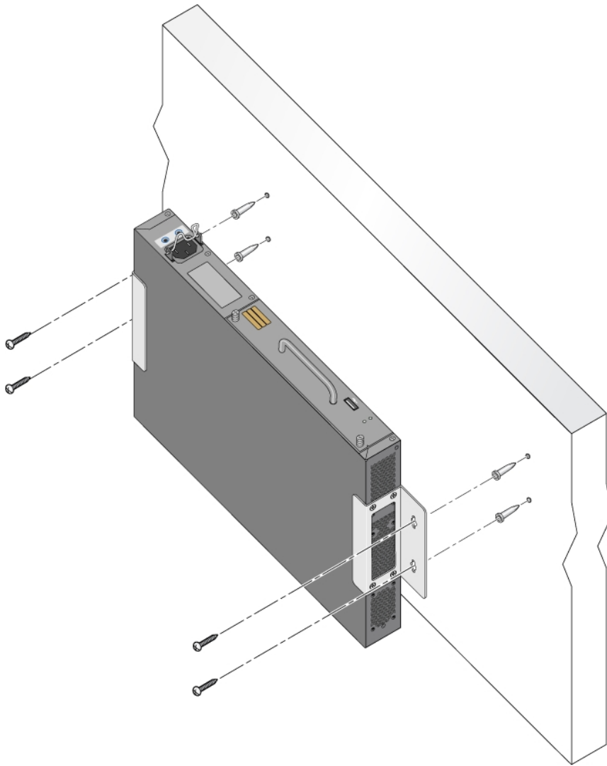
圖 13: 壁式安裝
