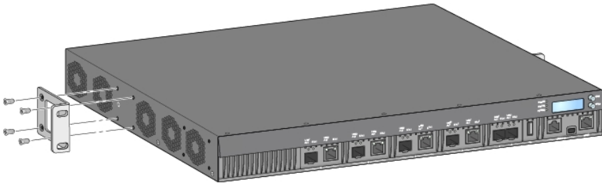
圖 9: 安裝中部安裝托架
