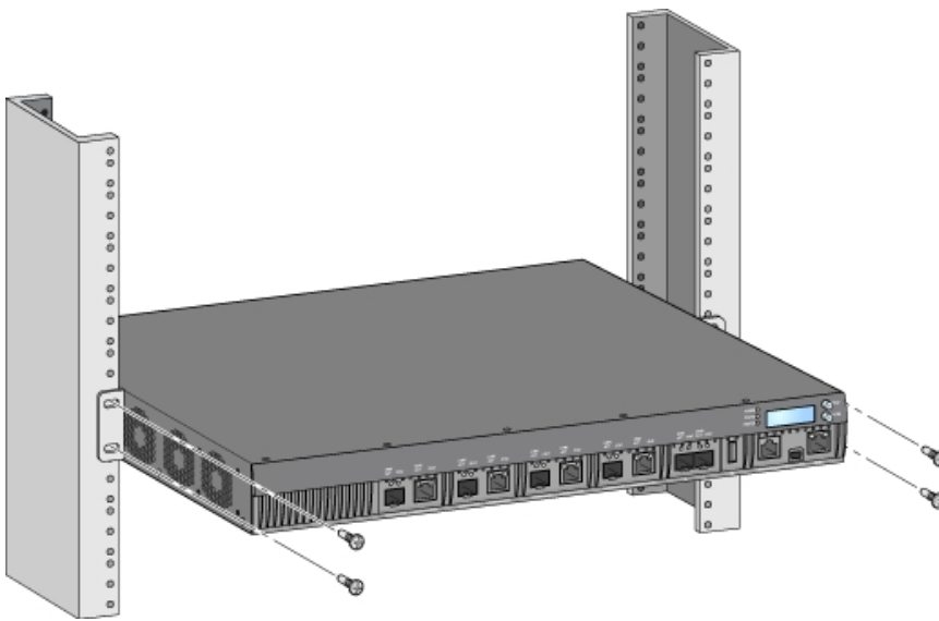
圖 10: 中部機架安裝
