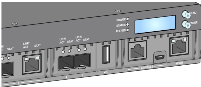
圖 4: 10GBASE-X 埠和 LED
