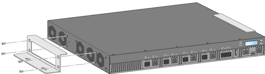
圖 12: 安裝壁式安裝托架
