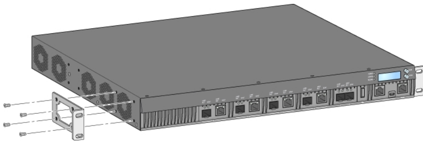
圖 7: 連接安裝托架
