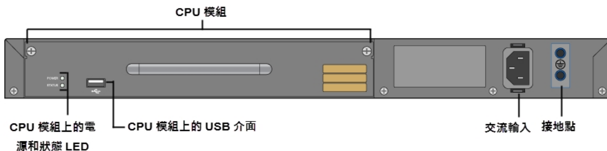
圖 2: W-7205 控制器的後置面板
